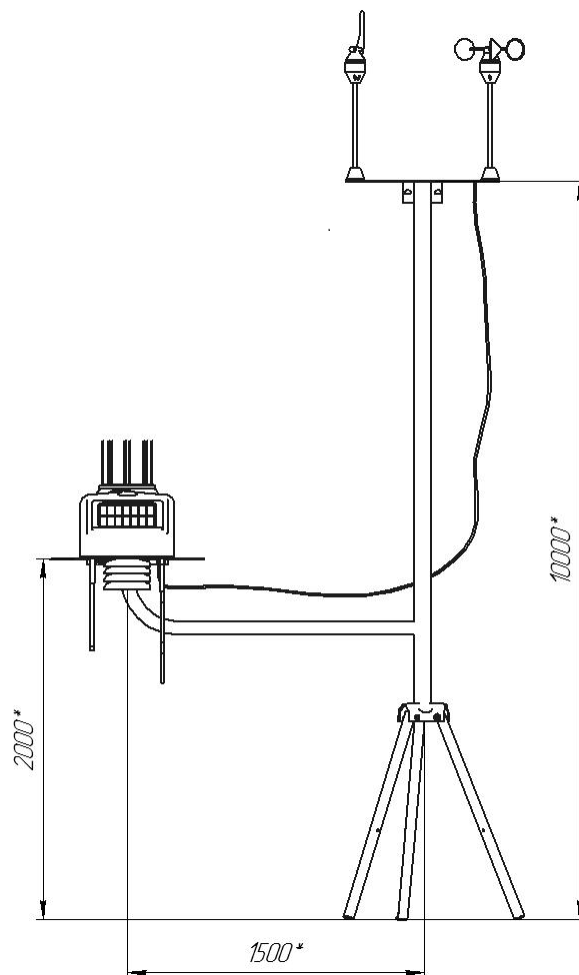
Рисунок 6 - Возможное расположение датчика ветра относительно метеостанции «СОКОЛ-М1»
