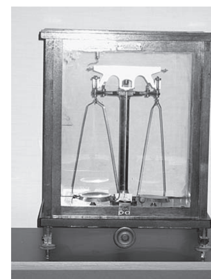
Аналитические весы, привезенные в эвакуацию, использовались в учебном процессе на кафедре агрохимии (изготовитель: магистр фармации Д. М. Генкель)
