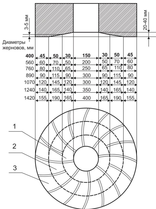
Рис. 6. Разбивка рабочей поверхности жернова:
