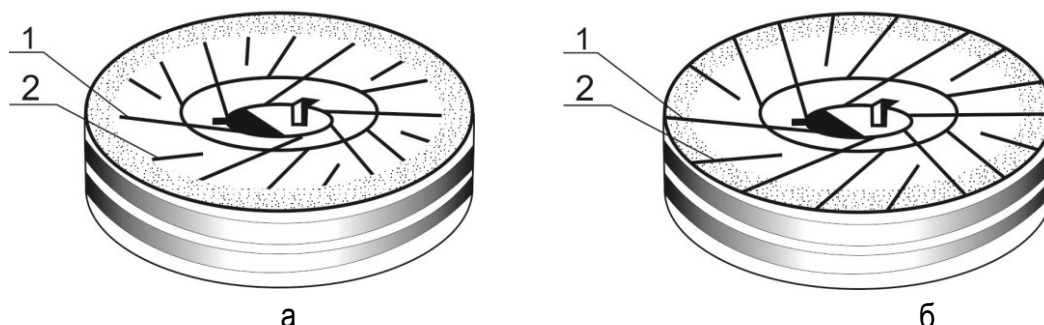
Рис. 5. Прямолинейные бороздки: а – для мельницы горизонтальной осью вращения, б – для мельницы вертикальной осью вращения; 1 – бороздка главная, 2 – бороздка второстепенная
