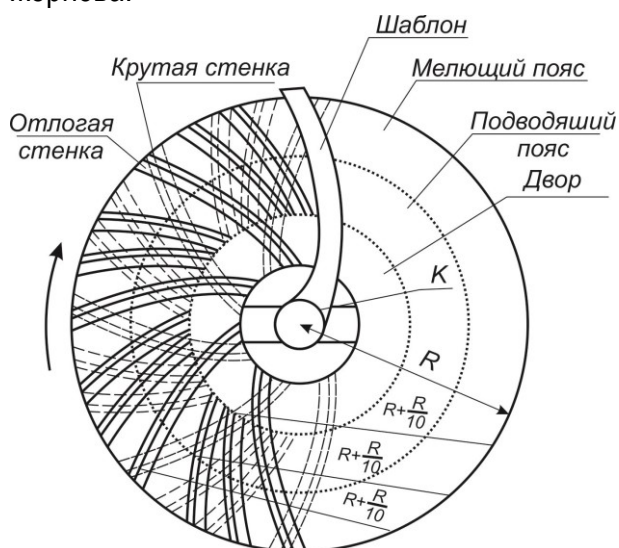
Рис. 4. Нанесение круговых бороздок на поверхности жерновов
