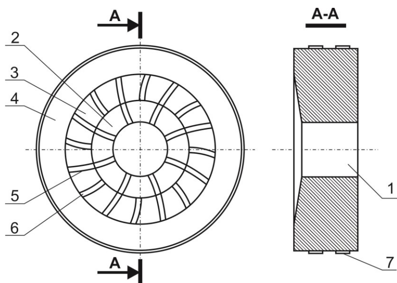
Рис. 1. Жерновые камни для мельницы с горизонтальной осью вращения, разбивка рабочей поверхности жернова:
