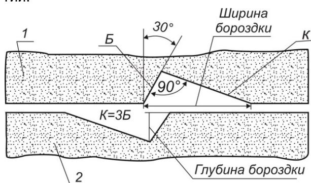
Рис. 3. Поперечное сечение бороздки: 1 – верхний камень, 2 – нижний камень; Б – крутая стенка, К – отлогая стенка
