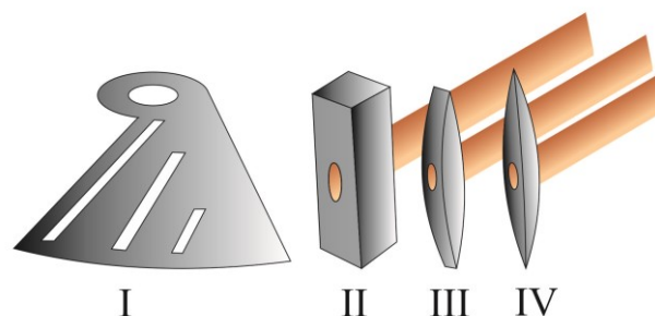
Рис. 7. Инструмент для насечки жерновов: I – шаблон; II – рязчик; III – насека; IV – клевец
