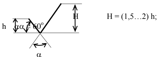
Рисунок 5.5 – Размеры условного знака
