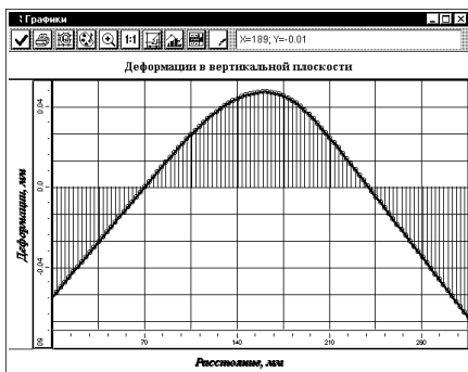
Рисунок 4.8 – Эпюра
