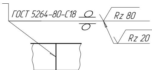
Рисунок 5.1 – Условное обозначение стыкового сварного шва
