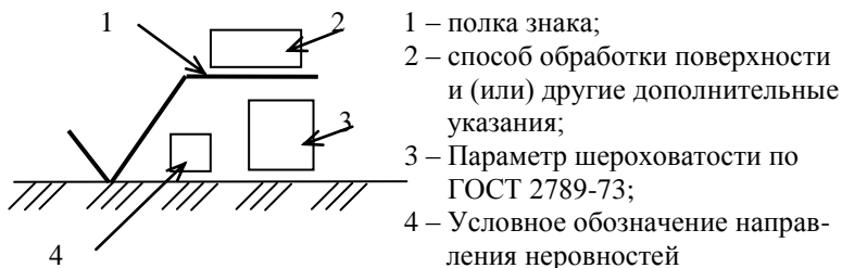
Рисунок 5.4 – Условный знак обозначения шероховатости поверхности
