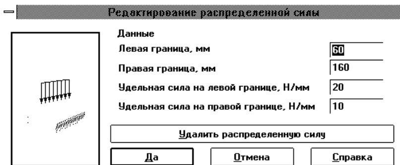
Рисунок 4.2 – Диалоговое окно для ввода и редактирования распределенных сил
